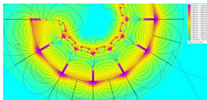
〔磁場解析によるマグネット配列検討〕
